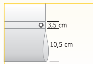
Detail Hohlraum-Konfektion
